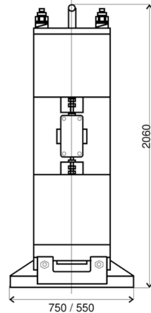
Enclume rectangulaire
